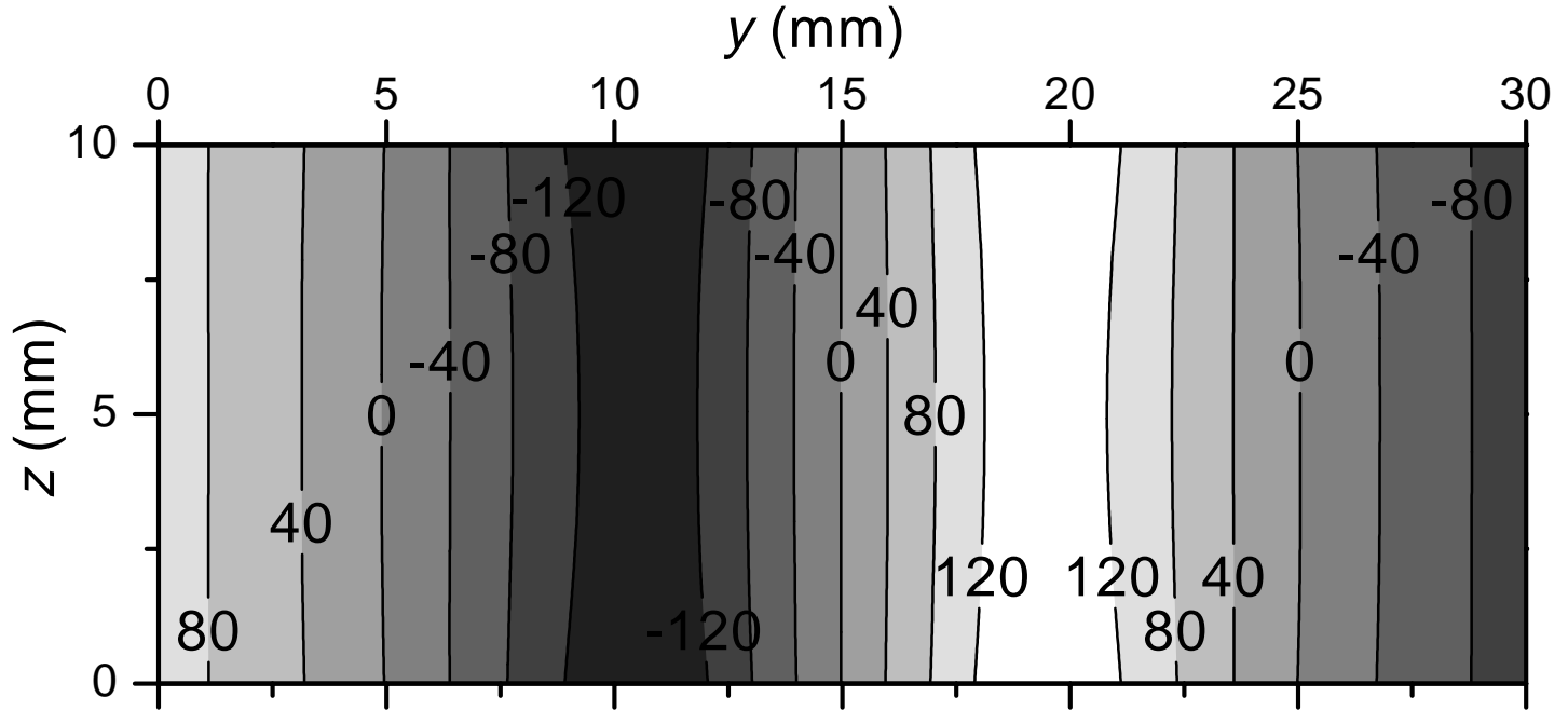
a. Bend test prediciton.
